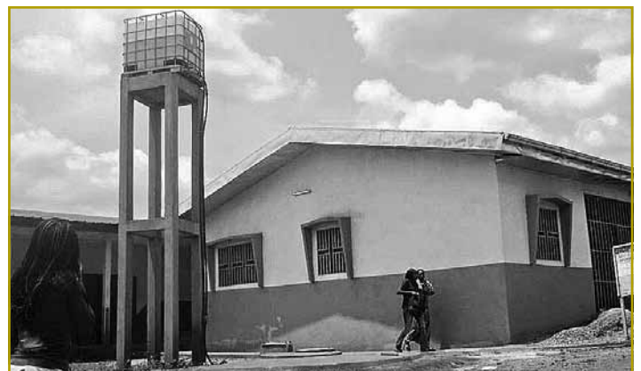
Blick auf die installierte Saugpumpe und den Wasserturm
